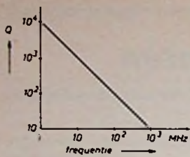
Fig. 4. Variatie van Q met de frequentie.
